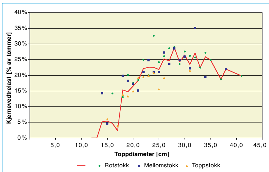
Figur 4: Utfallet av kjernevedtrelast. (Prispåslag 20 %, kjernevedkant > 80 %)
