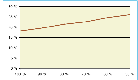
Figur 3: Utfall av kjernevedtrelast (y-aksen) som funksjon av kjernevedkant (x-aksen)
